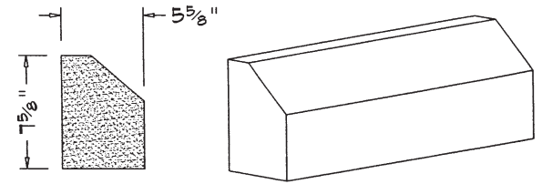
SL-232 (@ 23 5/8")
