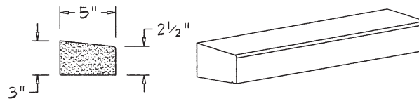
SL-240 (@ 36")
